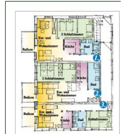
Grundriss Wohnung 1 bis 3
